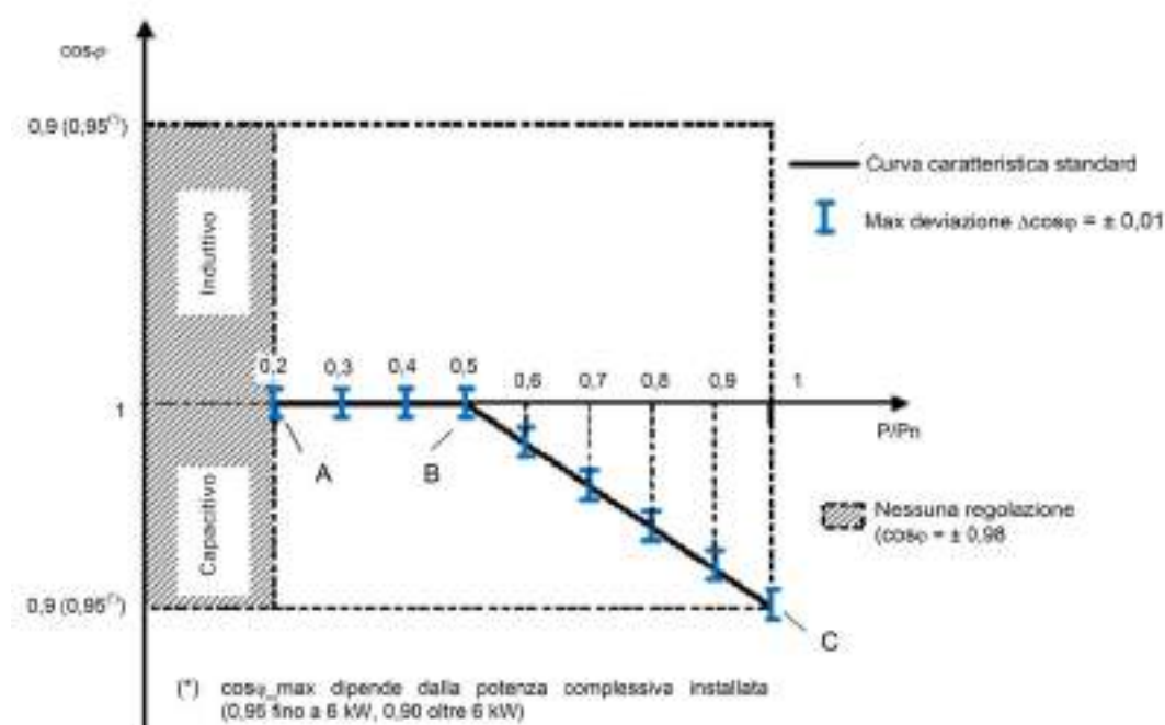
Figura 7Bbis – Curva caratteristica standard \cos\varphi = f(P)
