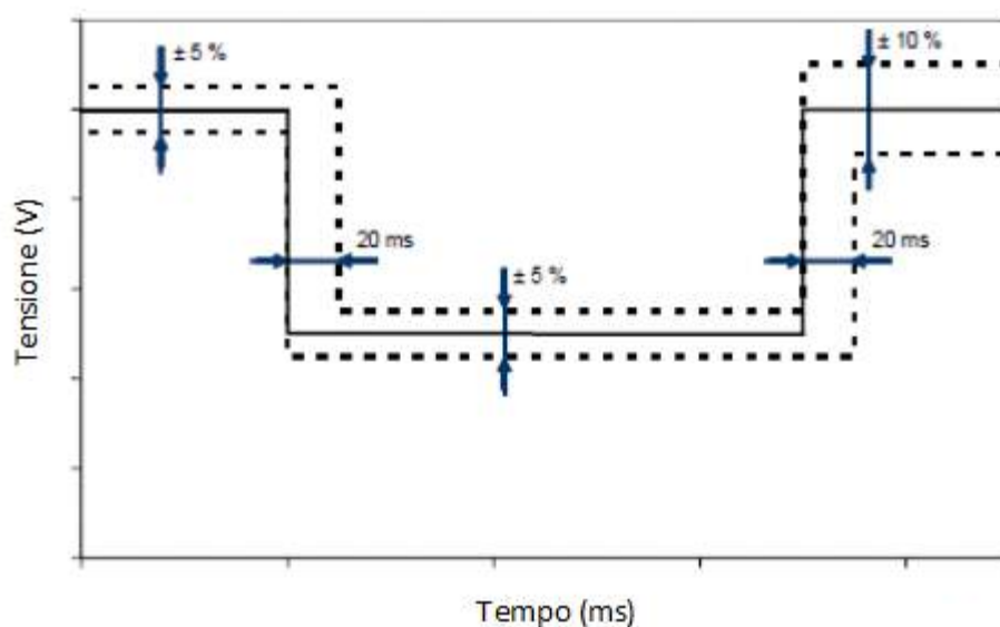
Figura 14Bbis – Tolleranze di ampiezza e tempo per le sequenze di prova di abbassamento della tensione di rete (VRT Test) (Fonte: norma IEC 61400-21, ed.2 – 2008/08)
