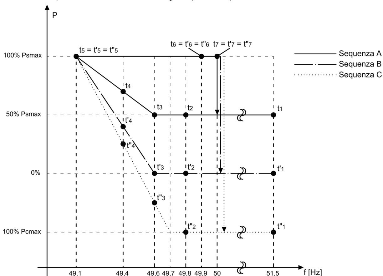
Figura 11Bbis – Curve di limitazione della potenza attiva
