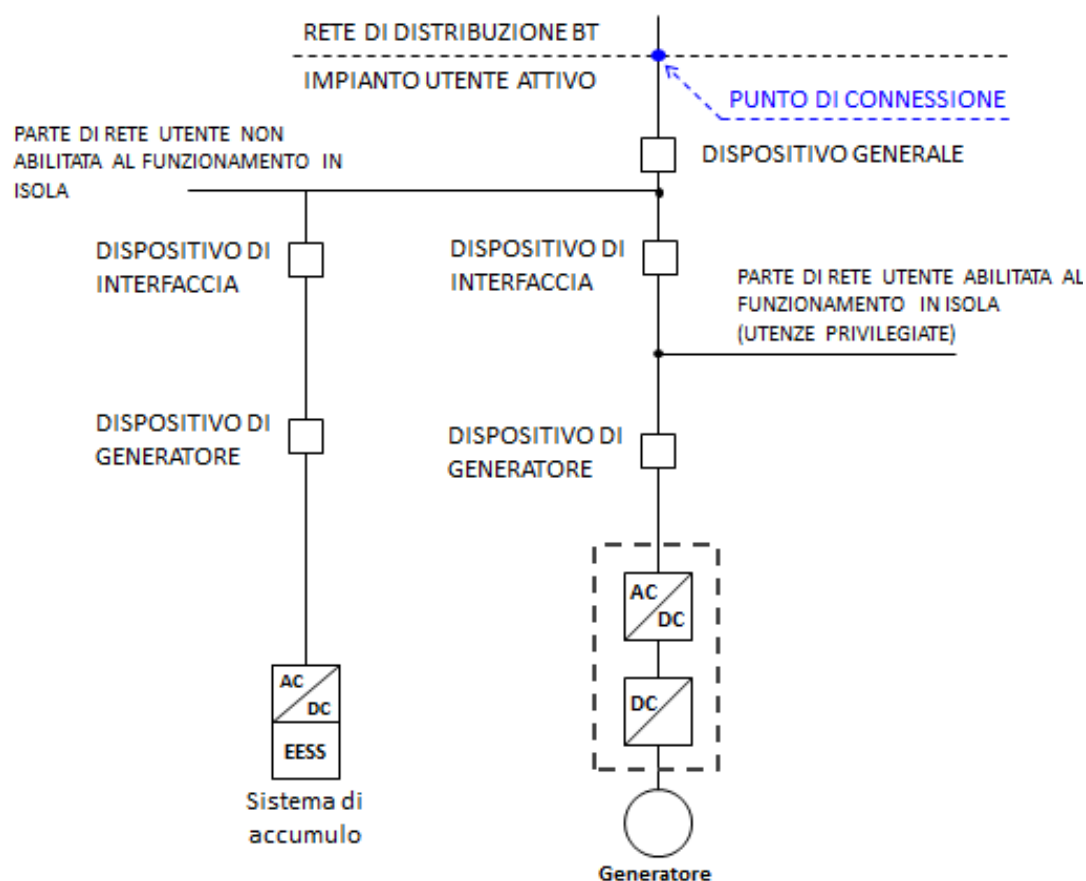
Figura 11d – Come in Fig. 10-c ma con sistema di accumulo posizionato nella parte di impianto in corrente alternata verso la parte di rete non abilitata al funzionamento in isola
