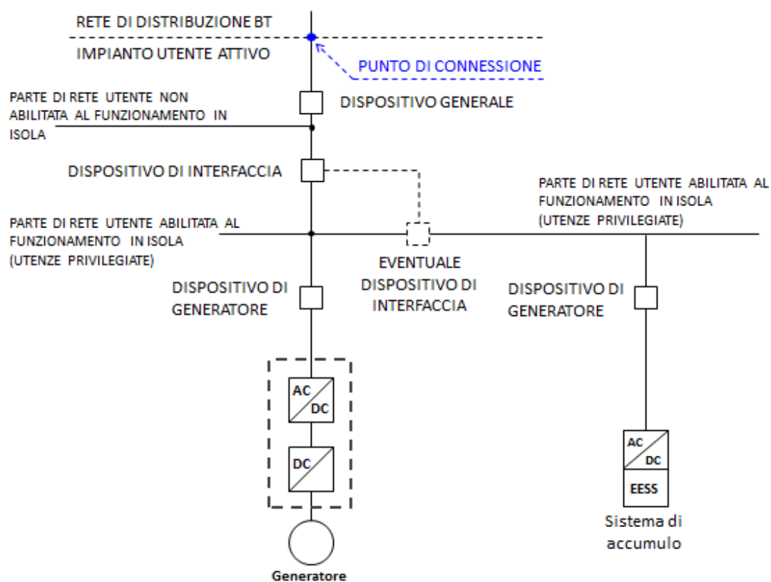
Figura 11c – Sistema di accumulo posizionato nella parte di impianto in corrente alternata a monte dell'inverter
