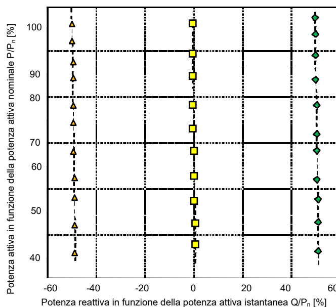
Figura 24 – Esempio di Grafico P(Q) . Massima potenza reattiva induttiva e capacitativa erogata in funzione della potenza attiva (qui è rappresentato il caso di un inverter di potenza superiore a 11,08kW, che deve poter assorbire o erogare a qualsiasi livello di potenza attiva una potenza reattiva pari almeno al 48,43 % della potenza attiva nominale, Q_{\min}/P_n = 48,43 \% P_n )
