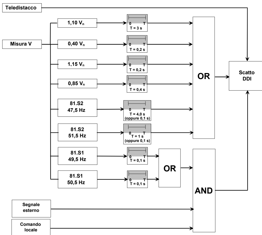
Figura 15 – Schema logico funzionale del SPI (i valori tra parentesi si riferiscono alla modalità transitoria di funzionamento del SPI)
