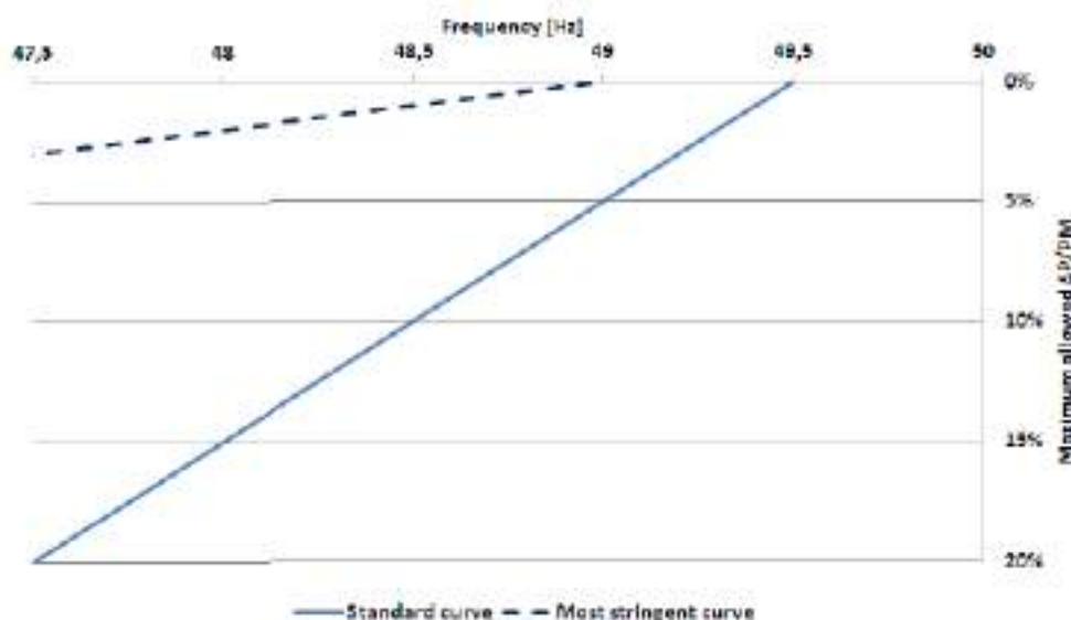
Figura 12bis – Riduzione della potenza attiva in regime di sottofrequenza
