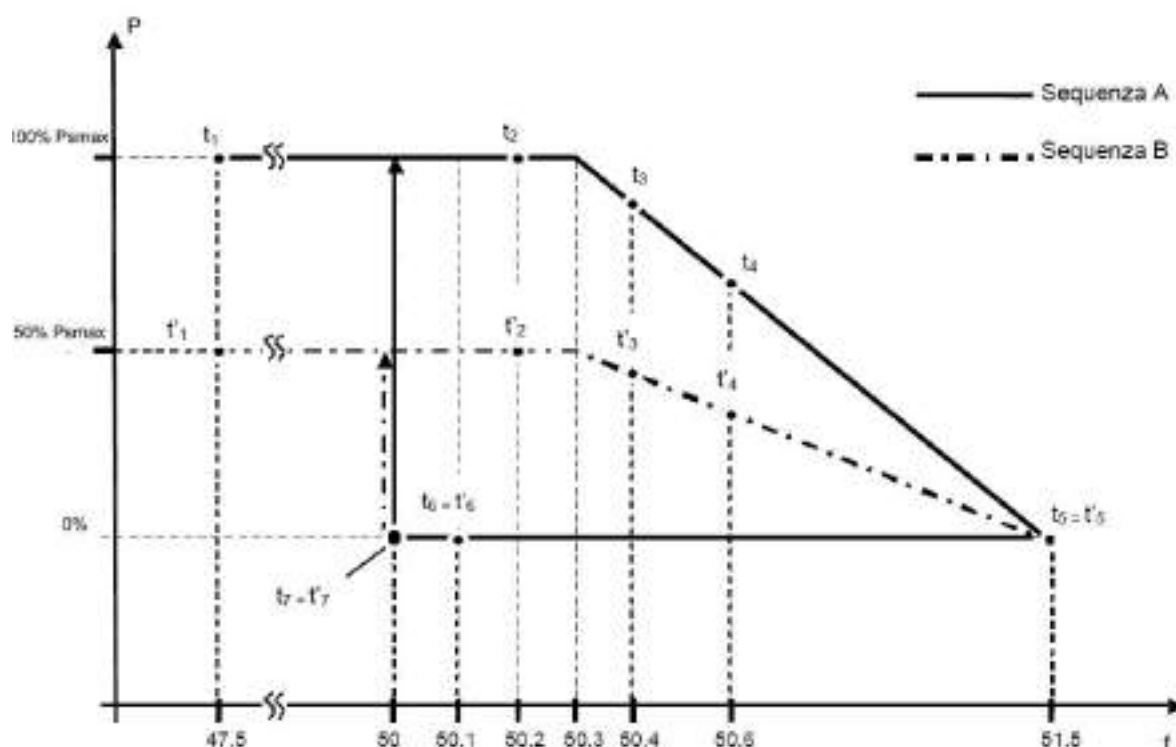
Figura 10Bbis – Curve di limitazione della potenza attiva per convertitori unidirezionali
