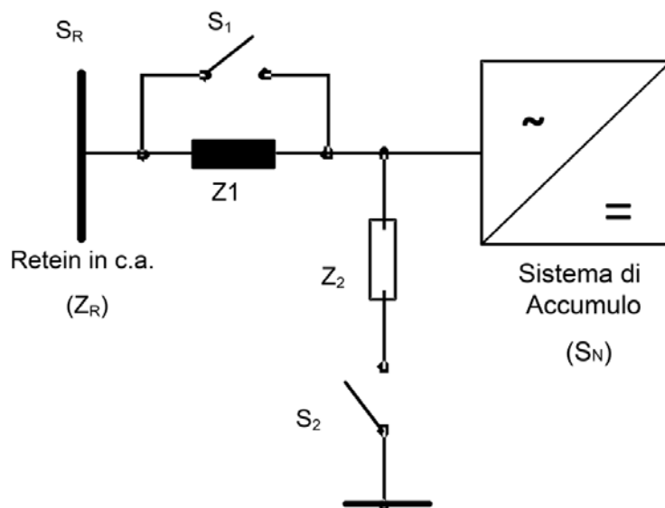
Figura 13Bbis – Esempio di circuito di prova per simulare gli abbassamenti temporanei di tensione
