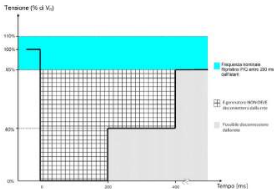
Figura 12Bbis – Requisiti per LVFRT.
