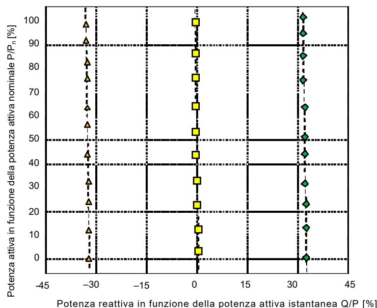
Figura 23 – Esempio di Grafico P(Q) . Massima potenza reattiva induttiva e capacitativa erogata in funzione della potenza attiva (qui è rappresentato il caso di un inverter di potenza fino a 11,08 kW, che deve poter erogare con un \cos\phi = 0,9 , ovvero Q/P = 0,4843 )
